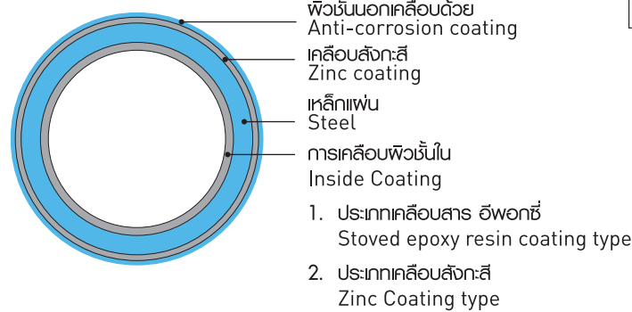
ภาพรูปตัดด้านข้างของท่อร้อยสายไฟฟ้า
