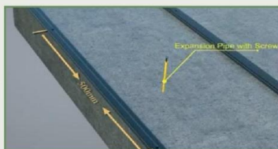
5. ติดตั้งชุดสกรูยึดโครงตรง บริเวณร่องตรงกลางของโครงตรง
