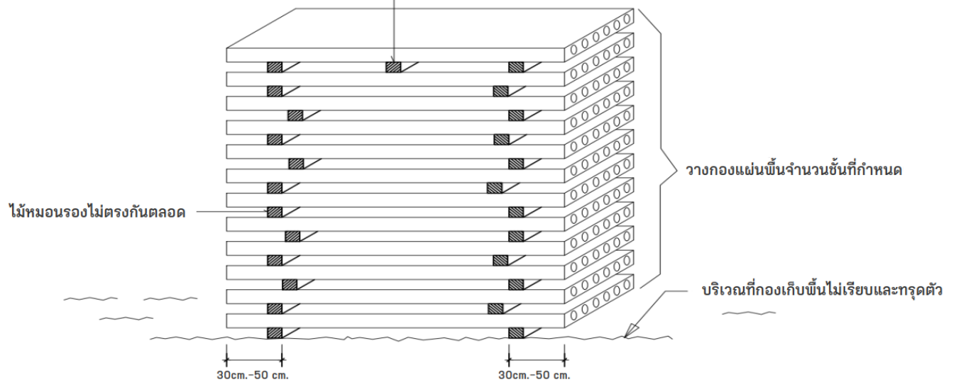
รูปที่ 5 แสดงวิธีลักษณะกองเก็บแผ่นพื้นที่ไม่ถูกต้อง
