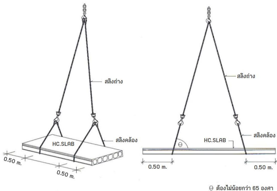
รูปที่ 10 แสดงลักษณะการคล้องสลิงเพื่อยกแผ่นพื้นฯ ที่ถูกต้อง
