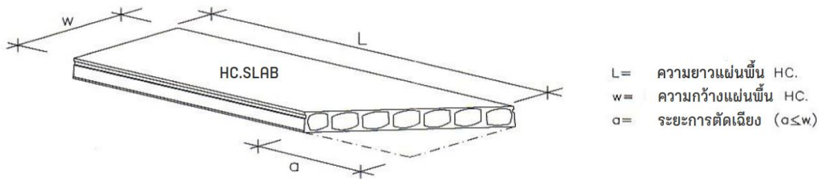
รูปที่ 22 แสดงการข้อกำหนดการตัดบากแผ่นเฉียง
