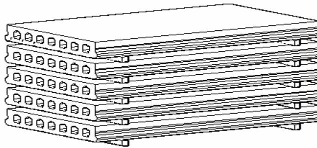
รูปที่ 30 แสดงการกองเก็บแผ่นพื้นฯที่ถูกต้อง
