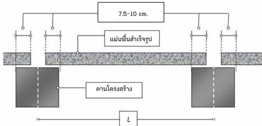
รูปที่ 11 แสดงระยะการวางแผ่นพื้นคอนกรีตสำเร็จรูปอัดแรงบนคานโครงสร้าง
