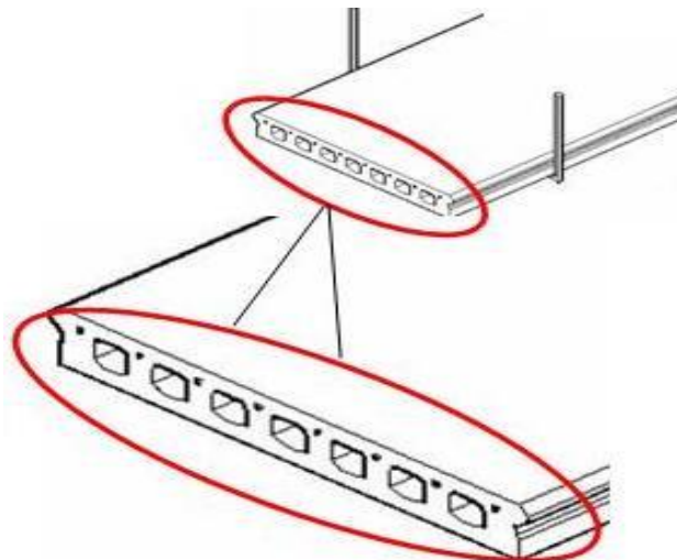
รูปที่ 29 แสดงการยกแผ่นพื้นในทิศทางที่ไม่ถูกต้อง
