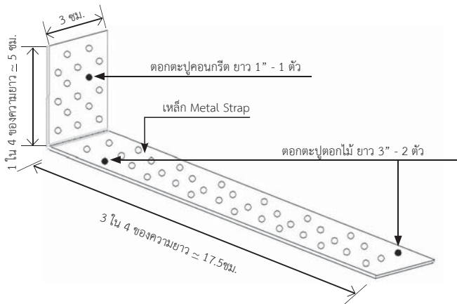
แบบขยาย Metal Strap
