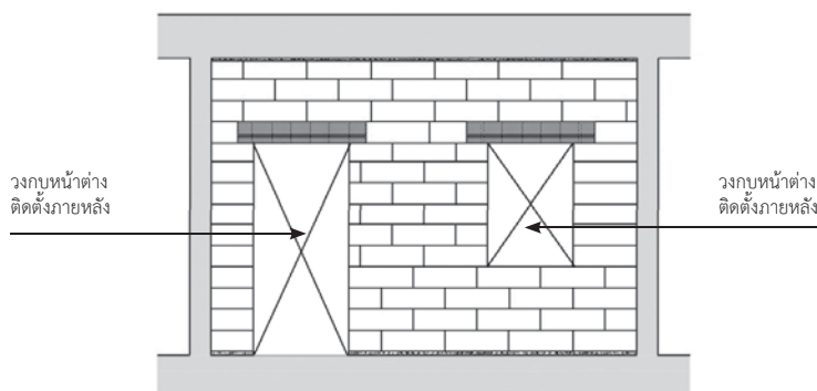
รูปการใช้คานกับหลังสำเร็จรูป (Lintel) สำหรับอิฐ Q-CON หนา 10 ซม.ขึ้นไป
