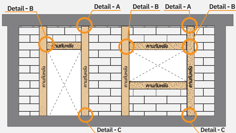
รูปการใช้คานกับหลังสำเร็จรูป สำหรับอิฐมวลเบา หนา 7.5 ซม.
