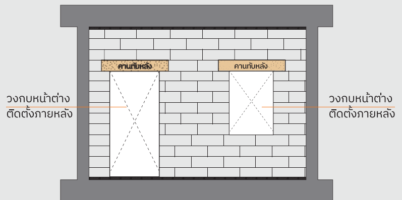
รูปการใช้คานกับหลังสำเร็จรูป สำหรับอิฐมวลเบา หนา 10 ซม.ขึ้นไป
