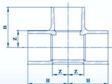
SIZE 125-300 mm
